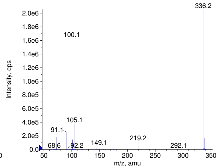
+ Oxeladin Prec(336.0) CE(99.0) RT(0.8)
