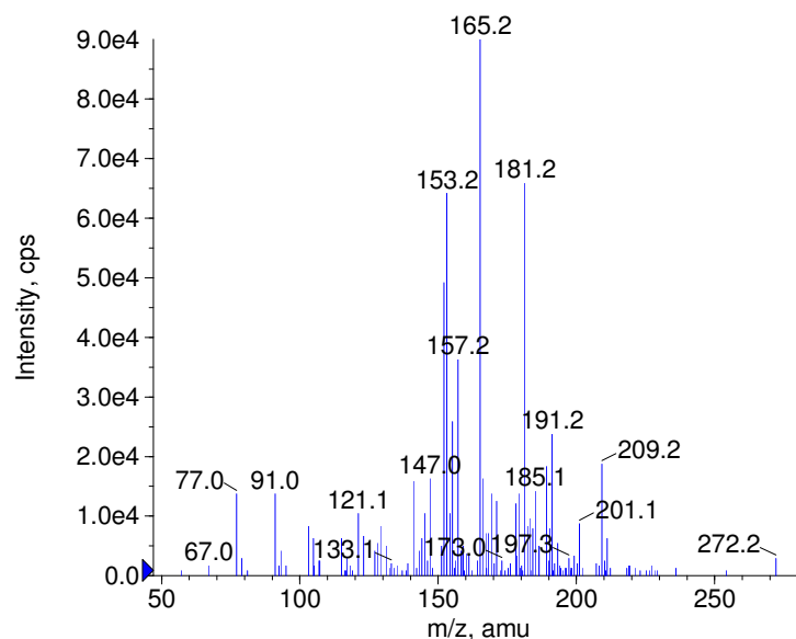
■ + Normorphine Prec(272.0) CE(50.0) RT(0.7)
