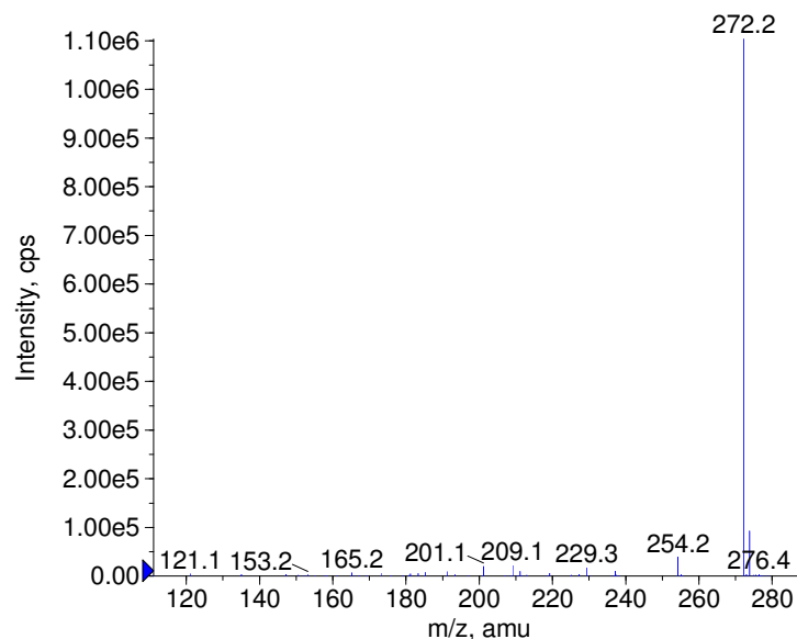
■ + Normorphine Prec(272.0) CE(50.0) RT(0.7)
