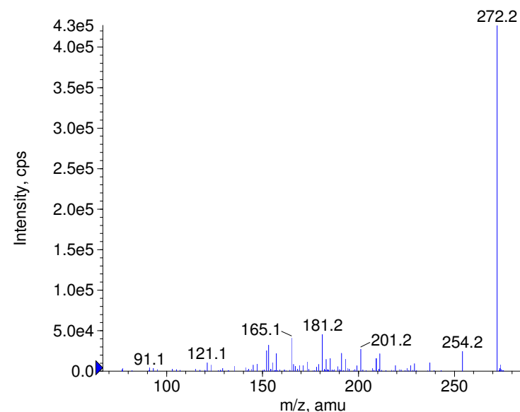
■ + Normorphine Prec(272.0) CE(99.0) RT(0.7)
