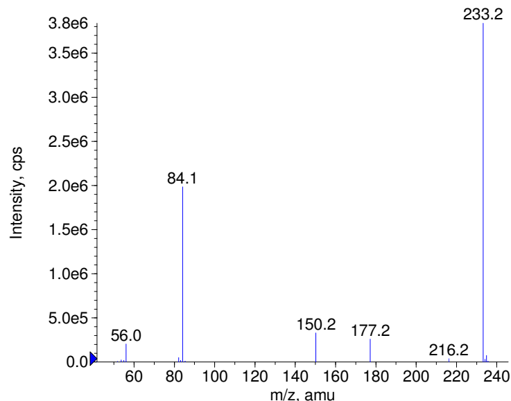
+ Norfentanyl Prec(233.0) CE(50.0) RT(0.9)
