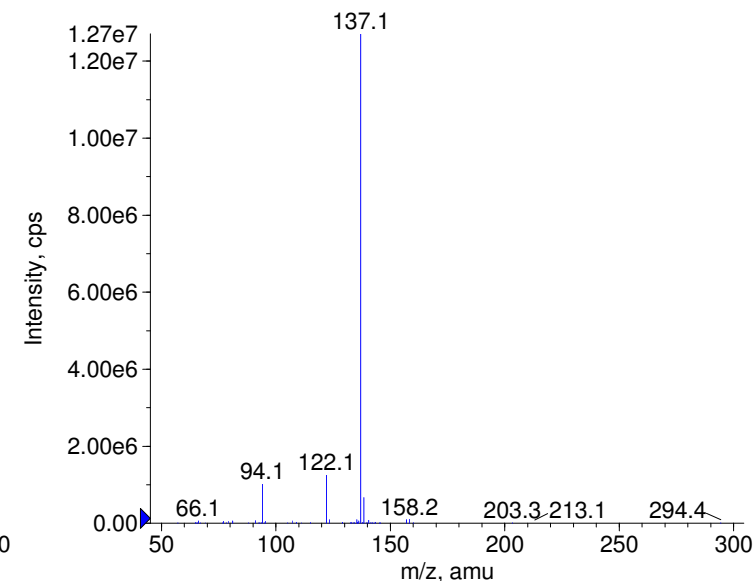
+ Nonivamide Prec(294.0) CE(99.0) RT(1.1)
