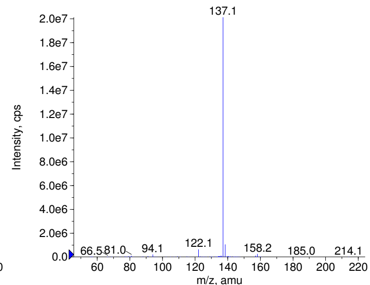
+ Nonivamide Prec(294.0) CE(99.0) RT(1.1)
