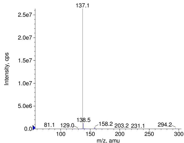
+ Nonivamide Prec(294.0) CE(50.0) RT(1.1)
