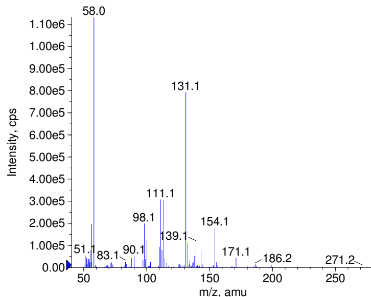
+ Nizatidine Prec(332.0) CE(50.0) RT(0.8)
