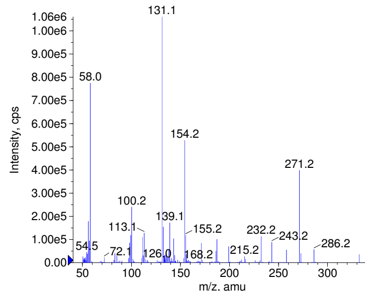
+ Nizatidine Prec(332.0) CE(99.0) RT(0.8)
