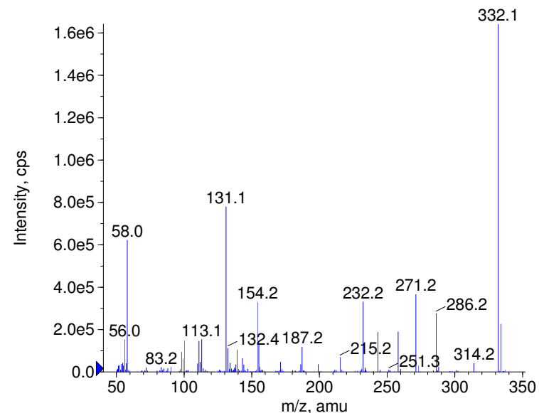
+ Nizatidine Prec(332.0) CE(99.0) RT(0.8)
