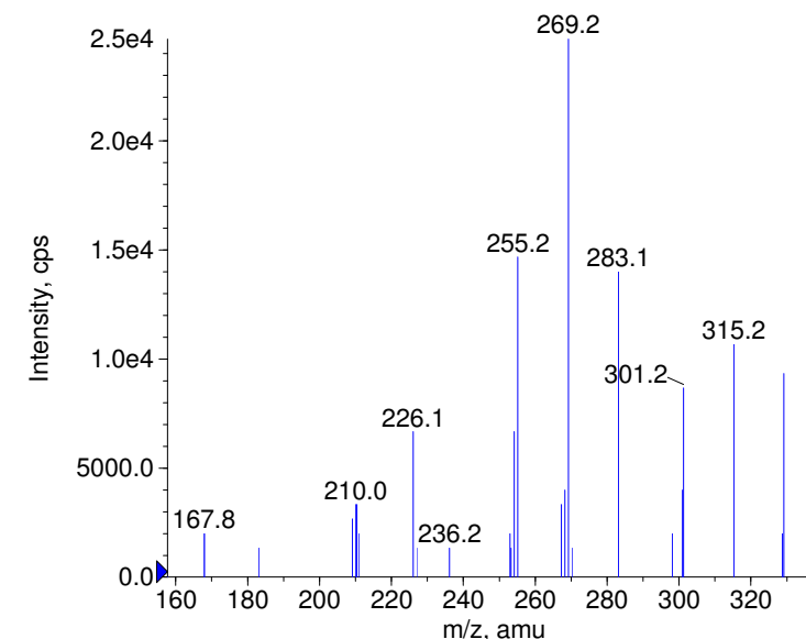
+ Nitrendipine Prec(361.0) CE(99.0) RT(0.8)
