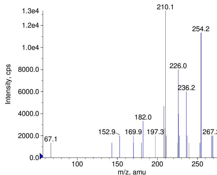
+ Nitrendipine Prec(361.0) CE(50.0) RT(0.8)
