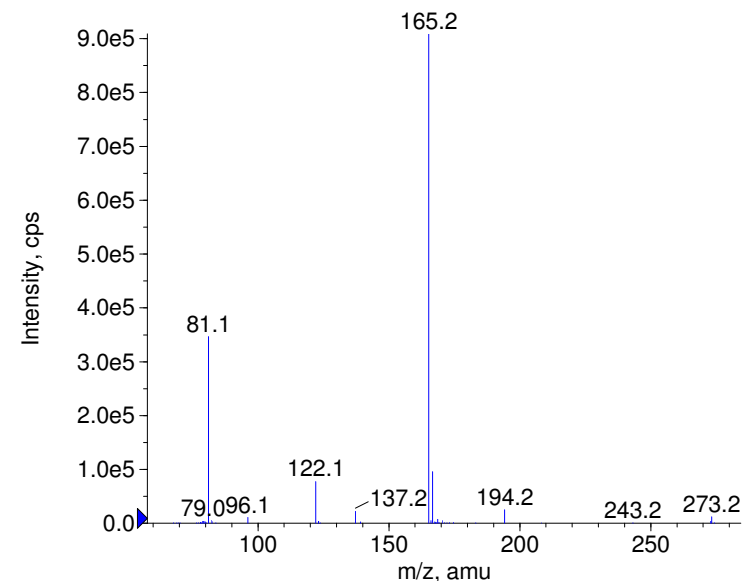
+ Nimustine Prec(273.0) CE(99.0) RT(0.8)
