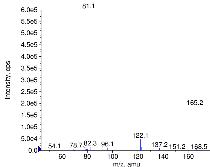
+ Nimustine Prec(273.0) CE(50.0) RT(0.8)
