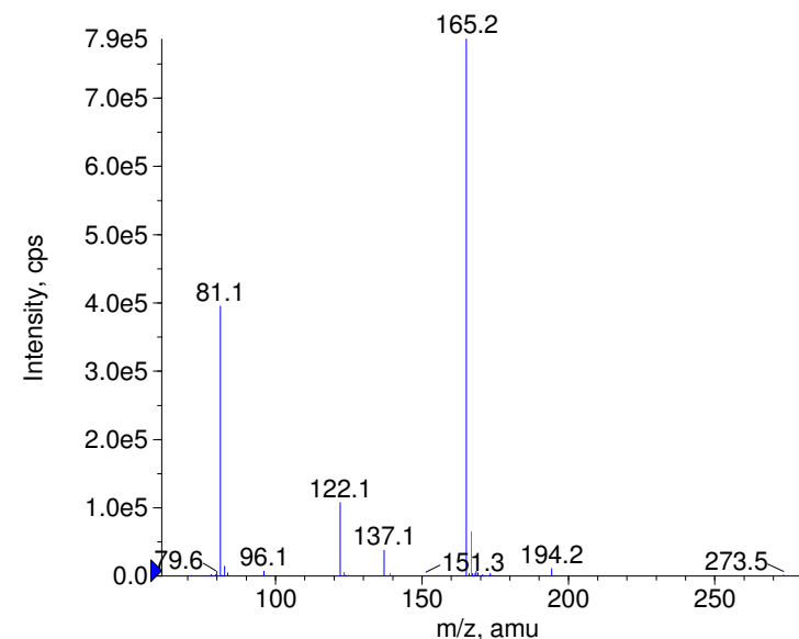
+ Nimustine Prec(273.0) CE(99.0) RT(0.8)
