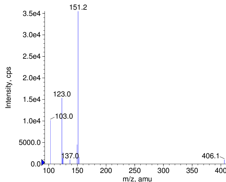
+ Nebivolol Prec(406.0) CE(50.0) RT(0.9)
