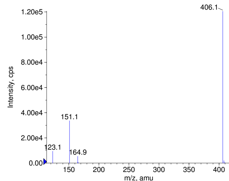
+ Nebivolol Prec(406.0) CE(99.0) RT(0.9)
