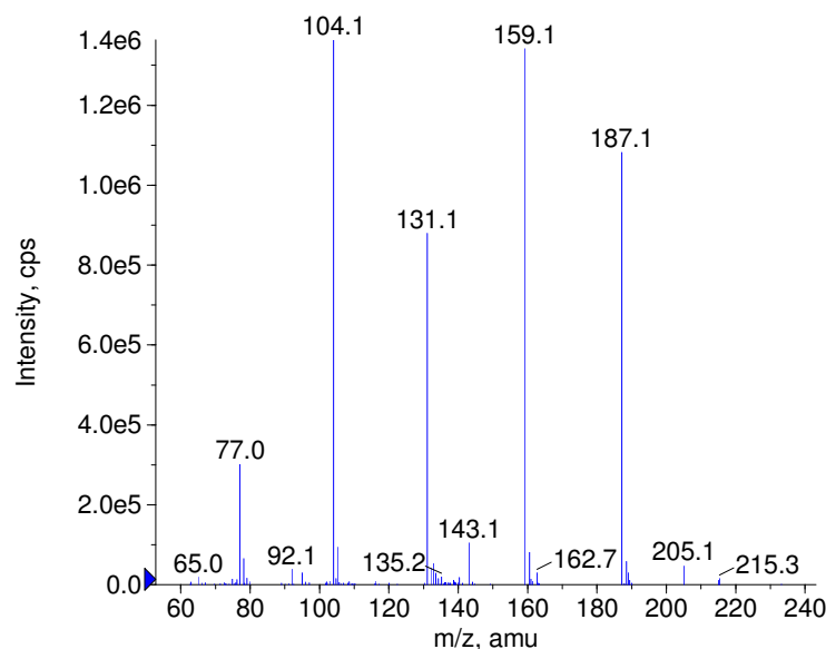
+ Nalidixic acid Prec(233.0) CE(50.0) RT(1.1)
