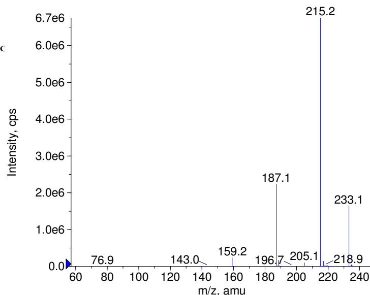
+ Nalidixic acid Prec(233.0) CE(50.0) RT(1.1)
