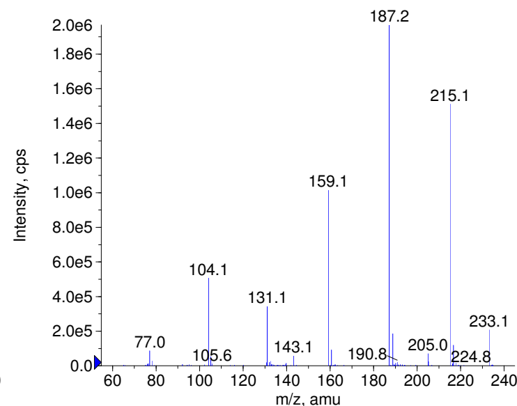
+ Nalidixic acid Prec(233.0) CE(99.0) RT(1.1)
