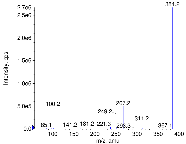
+ Naftidrofuryl Prec(384.0) CE(50.0) RT(0.7)
