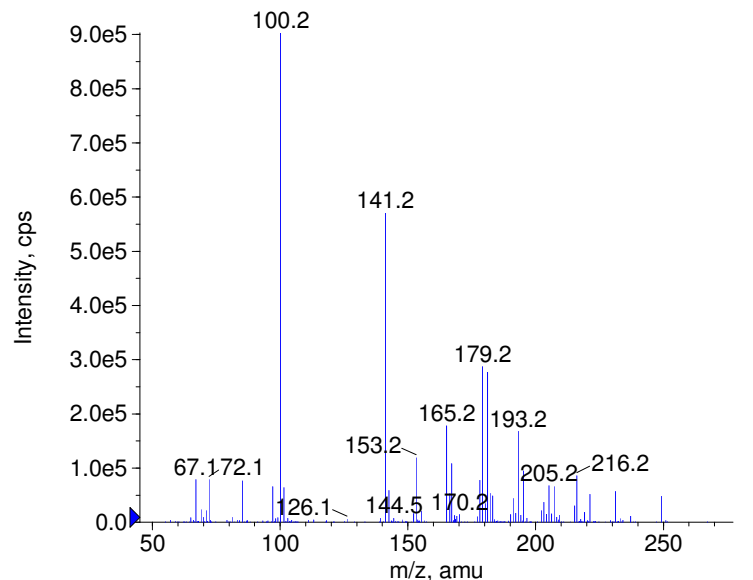
+ Naftidrofuryl Prec(384.0) CE(50.0) RT(0.7)
