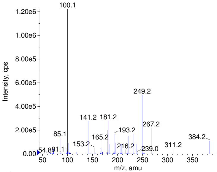
+ Naftidrofuryl Prec(384.0) CE(99.0) RT(0.8)
