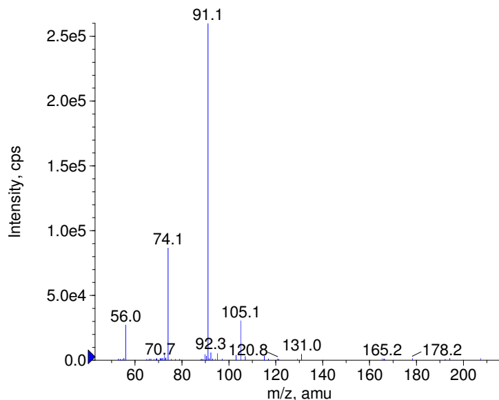
+ N-Despropylpropafenone Prec(300.0) CE(50.0) RT(0.8)
