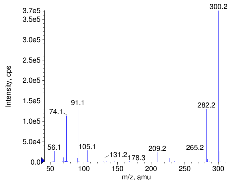
+ N-Despropylpropafenone Prec(300.0) CE(99.0) RT(0.8)
