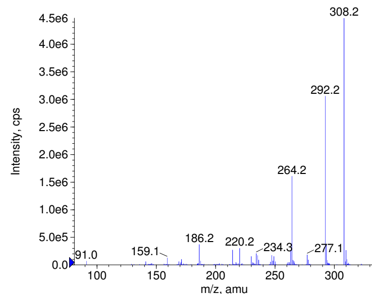
+ Moxaverine Prec(308.0) CE(99.0) RT(0.8)
