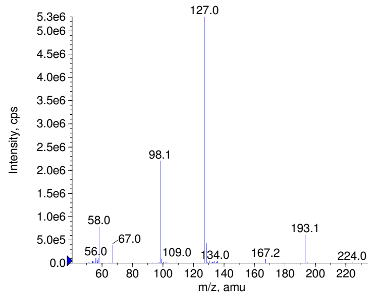
+ Monocrotophos Prec(224.0) CE(50.0) RT(0.9)
