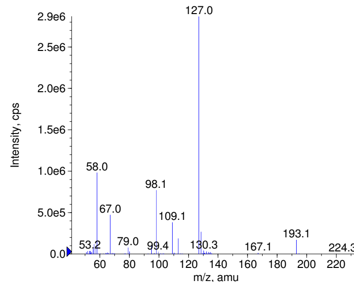
+ Monocrotophos Prec(224.0) CE(99.0) RT(0.9)
