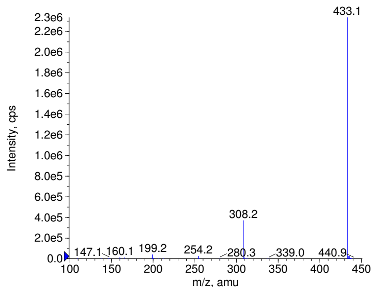
+ Mizolastine Prec(433.0) CE(50.0) RT(0.8)
