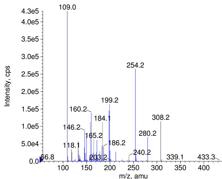
+ Mizolastine Prec(433.0) CE(50.0) RT(0.8)
