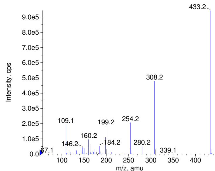
+ Mizolastine Prec(433.0) CE(99.0) RT(0.8)
