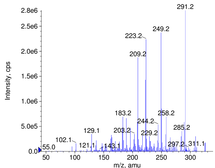
+ Midazolam Prec(326.0) CE(50.0) RT(0.8)
