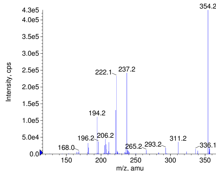
■ + Methysergide Prec(354.0) CE(99.0) RT(0.8)
