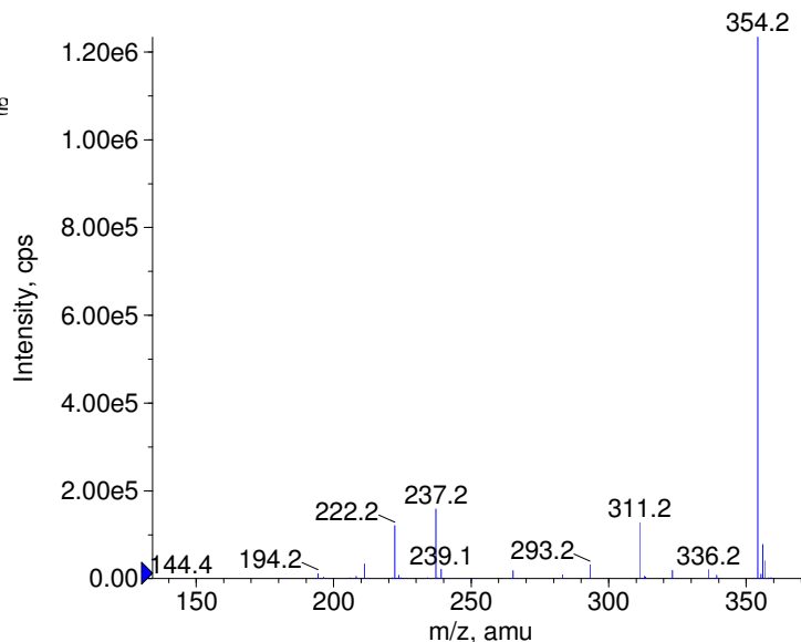
■ + Methysergide Prec(354.0) CE(50.0) RT(0.8)
