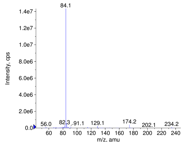
+ Methylphenidate Prec(234.0) CE(99.0) RT(0.9)
