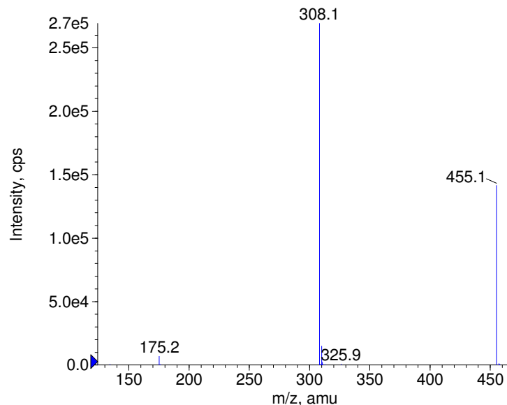
+ Methotrexate Prec(455.0) CE(50.0) RT(0.9)
