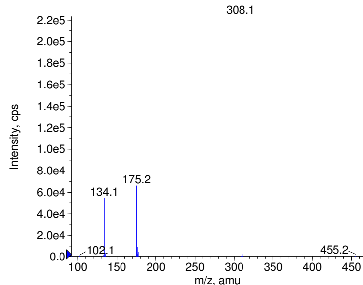
+ Methotrexate Prec(455.0) CE(99.0) RT(0.9)
