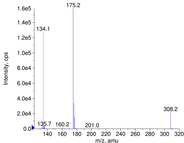
+ Methotrexate Prec(455.0) CE(50.0) RT(0.9)
