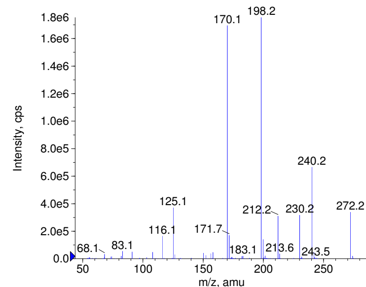
+ Methoprotryne Prec(272.0) CE(99.0) RT(1.0)
