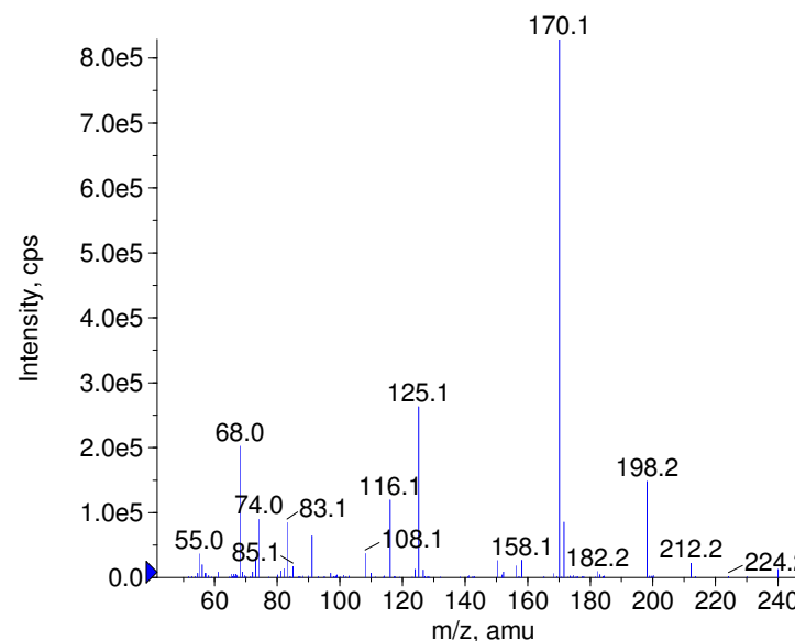
+ Methoprotryne Prec(272.0) CE(50.0) RT(1.0)
