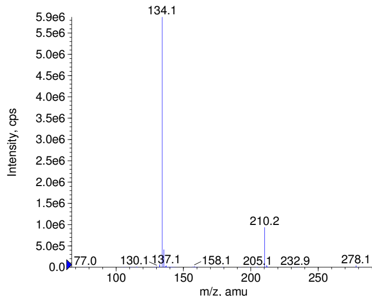
+ Metazachlor Prec(278.0) CE(50.0) RT(1.0)
