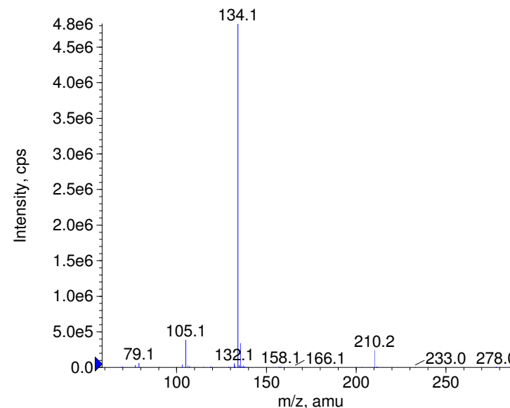
+ Metazachlor Prec(278.0) CE(99.0) RT(1.0)
