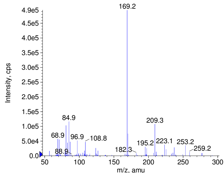
■ - Lincomycin Prec(405.0) CE(-50.0) RT(0.9)
