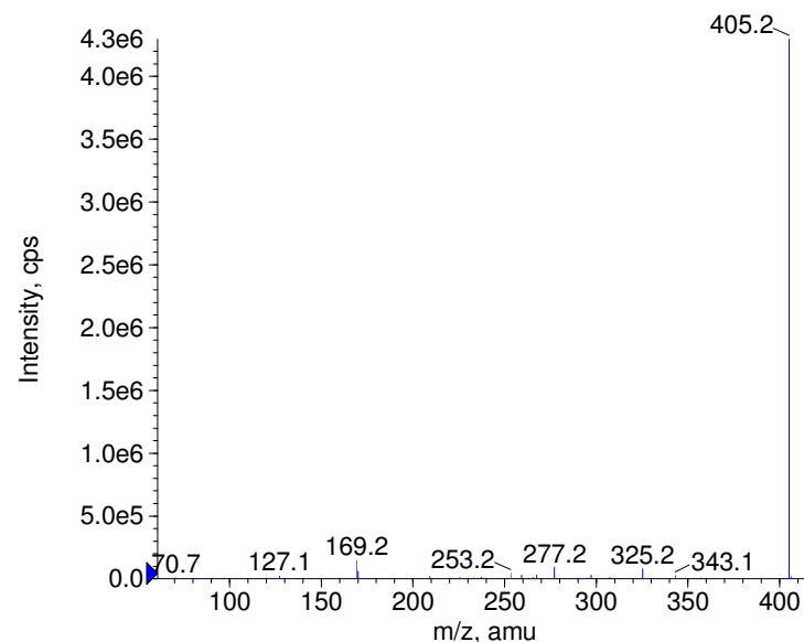
■ - Lincomycin Prec(405.0) CE(-50.0) RT(0.9)
