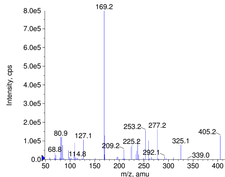
■ - Lincomycin Prec(405.0) CE(-99.0) RT(0.9)
