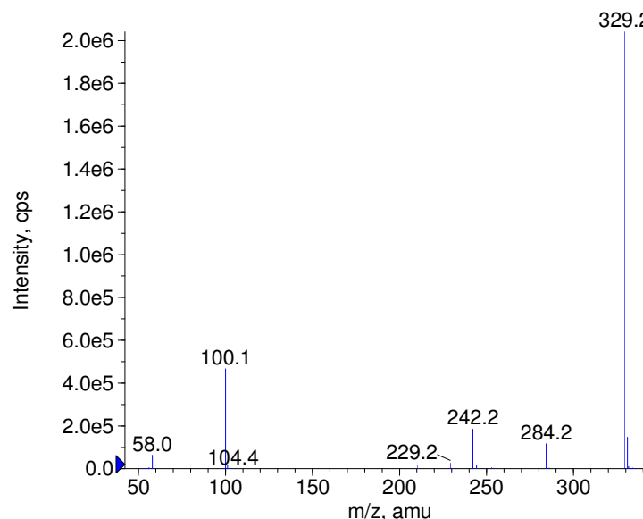
■ + Levomepromazine Prec(329.0) CE(50.0) RT(0.7)
