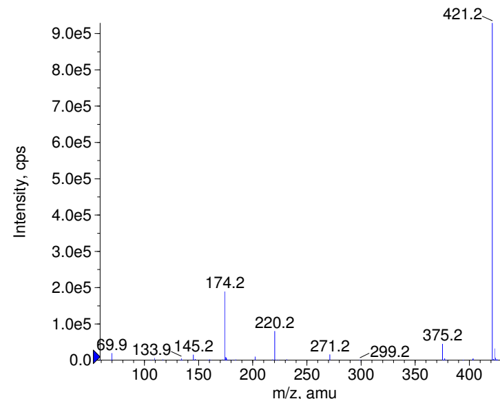
+ Levocabastine Prec(421.0) CE(99.0) RT(0.7)
