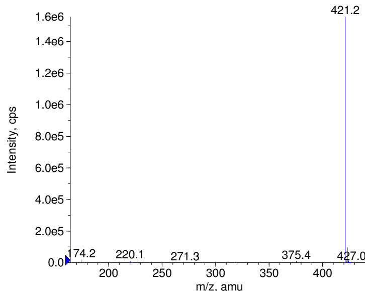
+ Levocabastine Prec(421.0) CE(50.0) RT(0.7)
