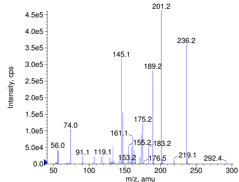
+ Levobunolol Prec(292.0) CE(99.0) RT(0.7)
