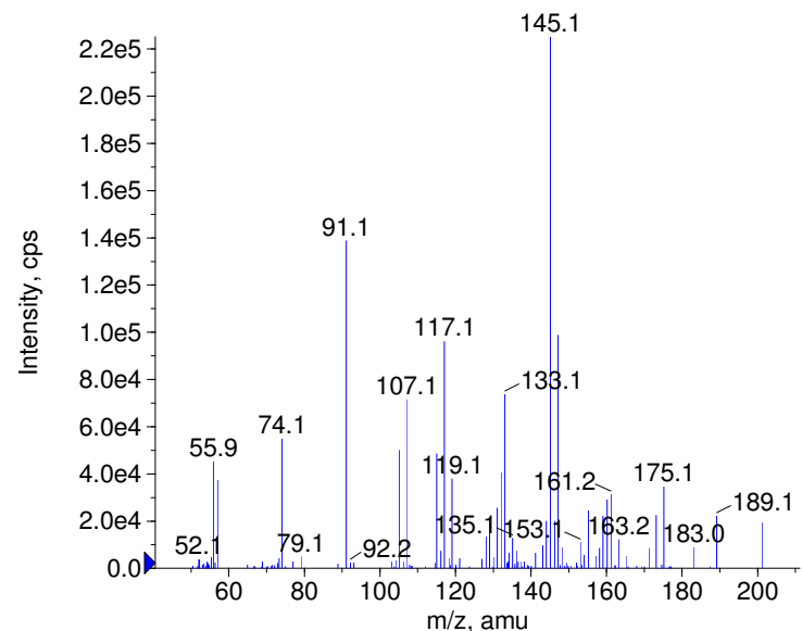
+ Levobunolol Prec(292.0) CE(50.0) RT(0.7)
