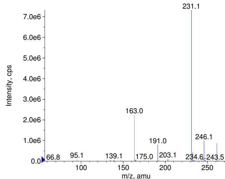
+ Khellin Prec(261.0) CE(99.0) RT(1.0)
