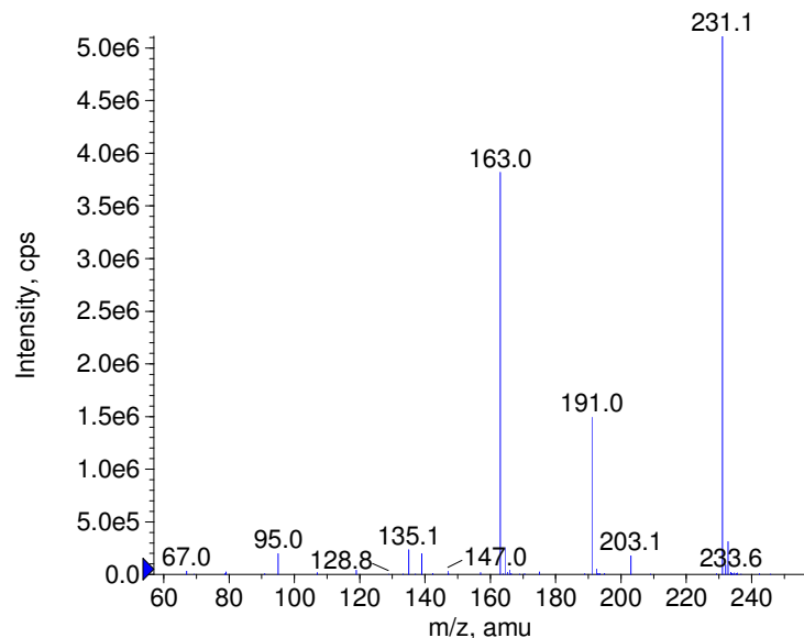
+ Khellin Prec(261.0) CE(50.0) RT(0.9)
