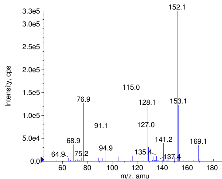
+ Kavain Prec(231.0) CE(50.0) RT(1.1)
