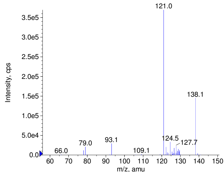
+ Isoniazide Prec(138.0) CE(50.0) RT(0.7)
