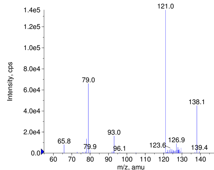
+ Isoniazide Prec(138.0) CE(99.0) RT(0.8)
