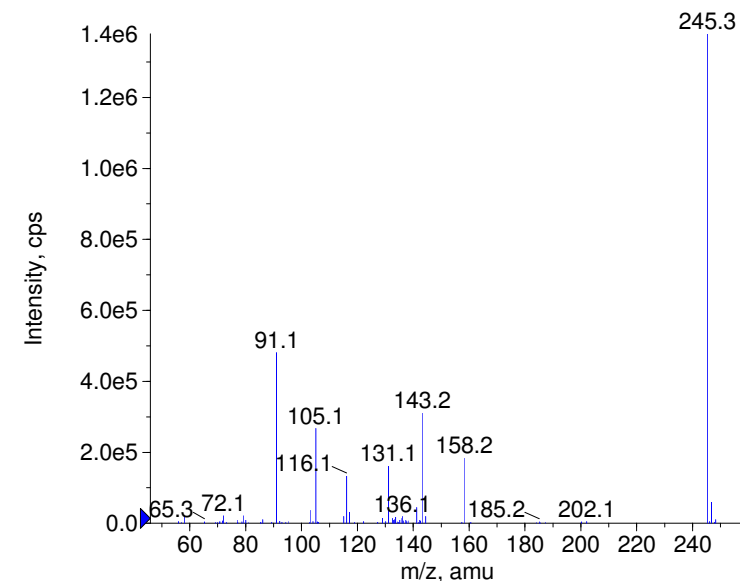
+ Isoaminile Prec(245.0) CE(99.0) RT(0.9)
