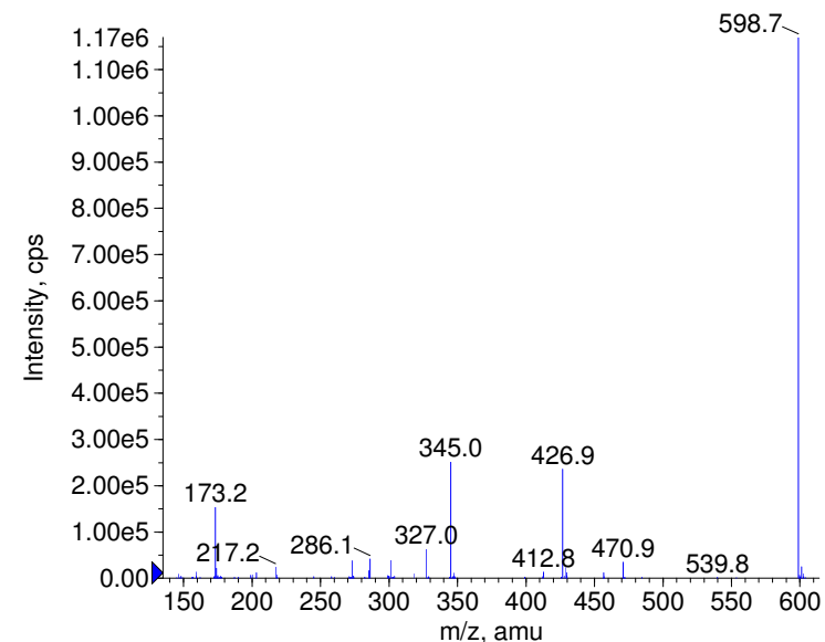
■ + Iopodic acid Prec(599.0) CE(99.0) RT(1.2)
