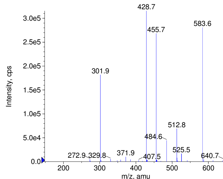
+ Ioglicic acid Prec(672.0) CE(99.0) RT(1.0)
