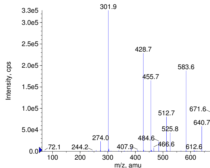
+ Ioglicic acid Prec(672.0) CE(99.0) RT(1.0)
