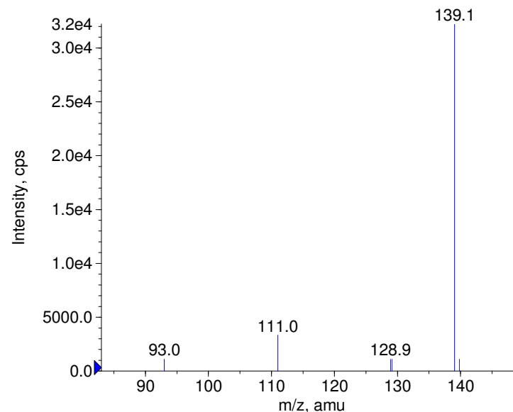
+ Indomethacin Prec(358.0) CE(50.0) RT(0.8)
