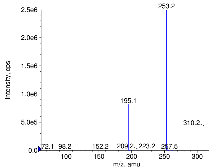
+ Hexobendine Prec(593.0) CE(50.0) RT(1.0)
