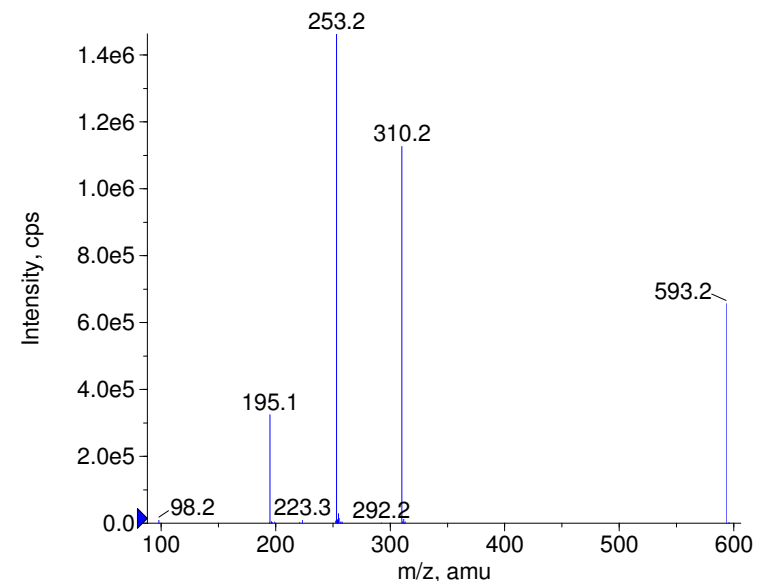
+ Hexobendine Prec(593.0) CE(99.0) RT(1.0)
