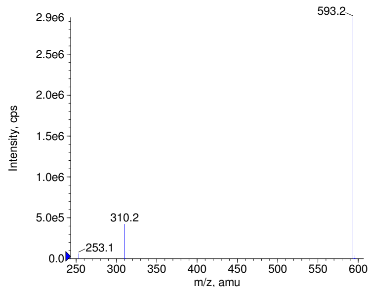
+ Hexobendine Prec(593.0) CE(50.0) RT(1.0)
