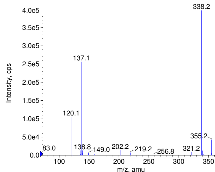
■ + Hexamidine Prec(355.0) CE(99.0) RT(0.8)
