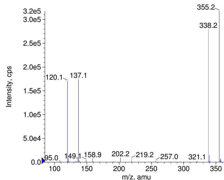
■ + Hexamidine Prec(355.0) CE(99.0) RT(0.8)
