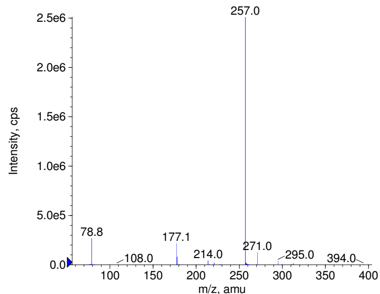
■ - Halofuginone Prec(412.0) CE(-50.0) RT(0.9)
