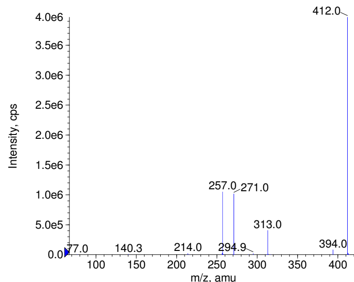
■ - Halofuginone Prec(412.0) CE(-50.0) RT(0.9)
