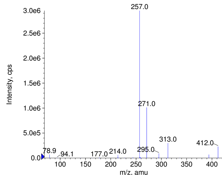
■ - Halofuginone Prec(412.0) CE(-99.0) RT(0.9)
