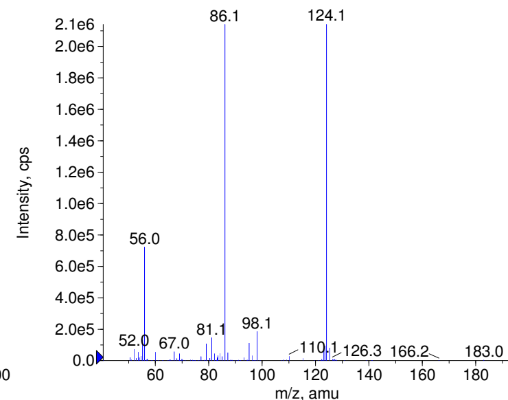
+ Guanacine Prec(183.0) CE(99.0) RT(1.6)
