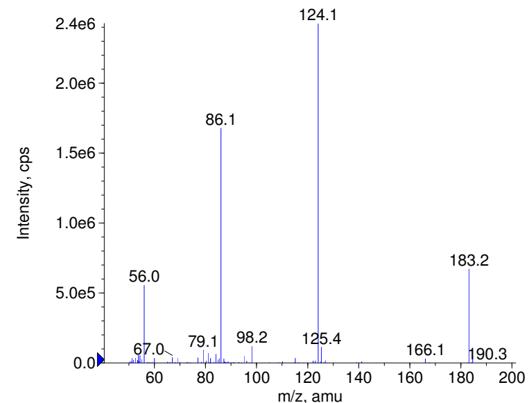
+ Guanacine Prec(183.0) CE(99.0) RT(1.6)
