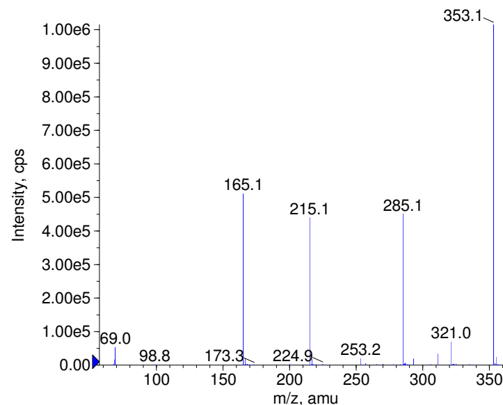
+ Griseofulvin Prec(353.0) CE(50.0) RT(1.2)
