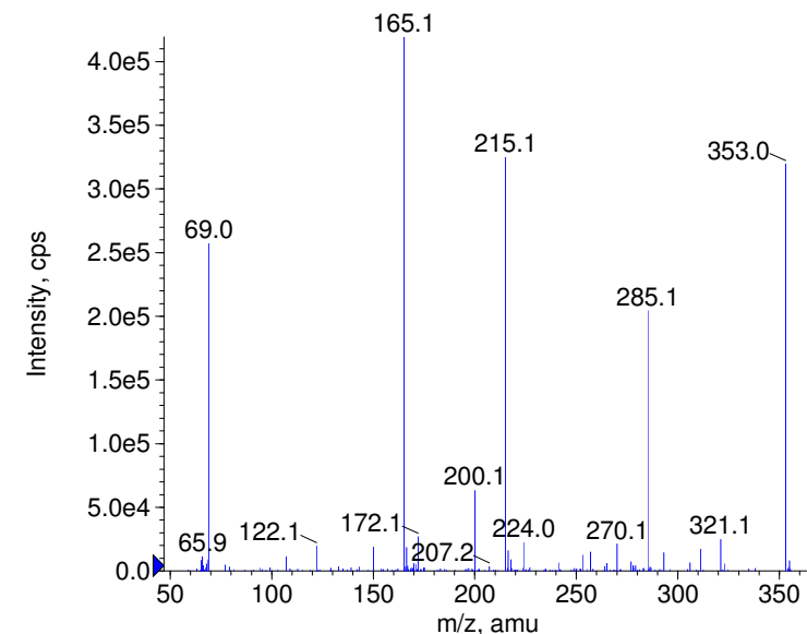
+ Griseofulvin Prec(353.0) CE(99.0) RT(1.2)
