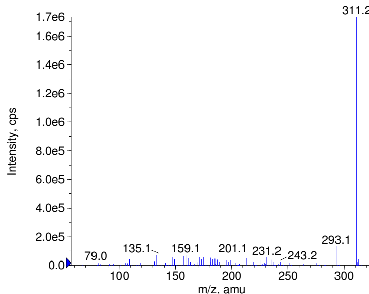
■ + Gestodene Prec(311.0) CE(50.0) RT(0.9)
