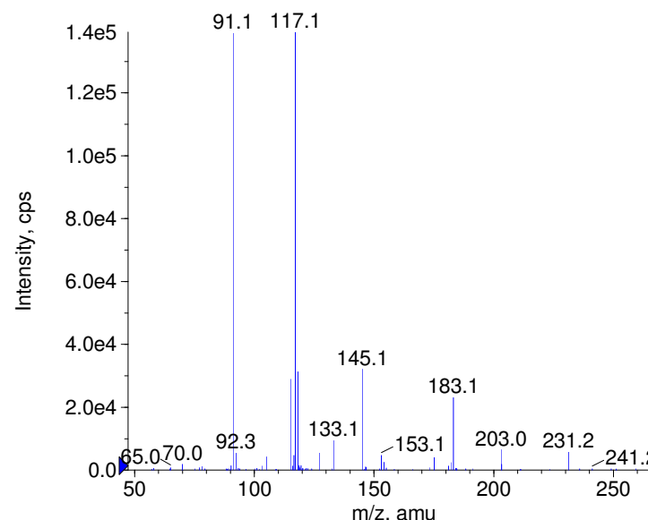
+ Fluoxetine Prec(310.0) CE(50.0) RT(1.0)
