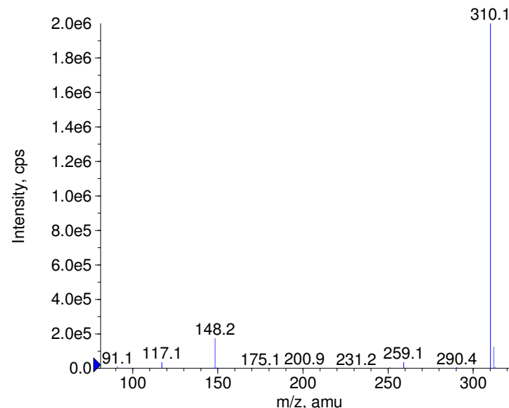
+ Fluoxetine Prec(310.0) CE(50.0) RT(1.0)
