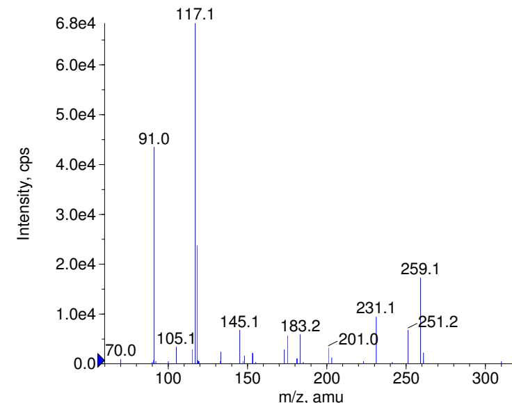
+ Fluoxetine Prec(310.0) CE(99.0) RT(1.0)
