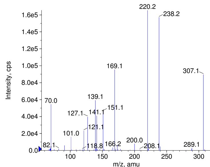
+ Fluconazole Prec(307.0) CE(99.0) RT(0.7)
