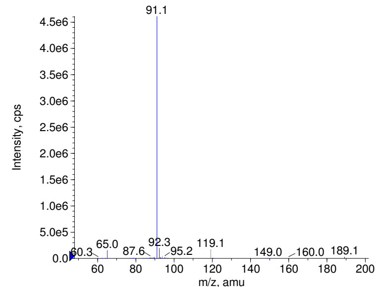
+ Fenproporex Prec(189.0) CE(99.0) RT(0.9)
