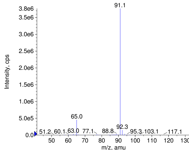
+ Fenproporex Prec(189.0) CE(50.0) RT(0.9)
