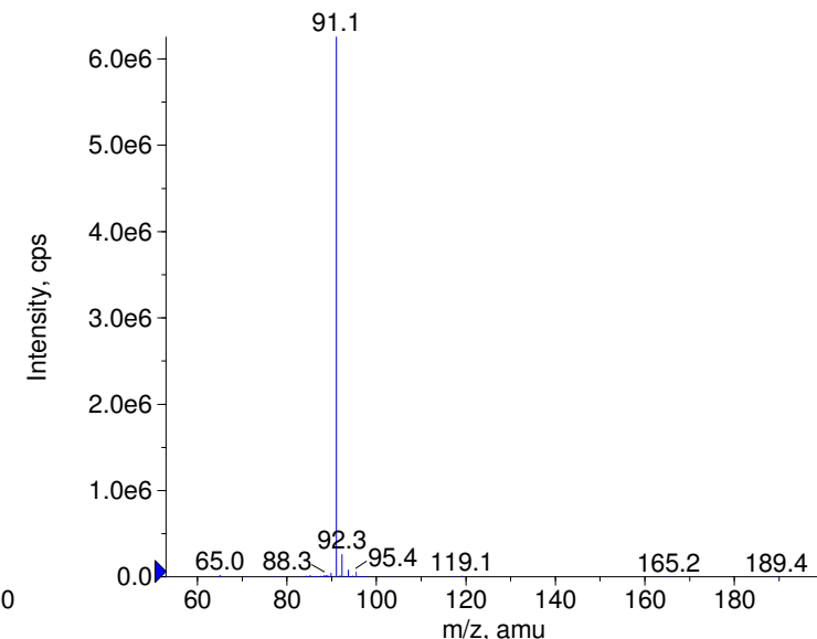
+ Fenproporex Prec(189.0) CE(99.0) RT(0.9)
