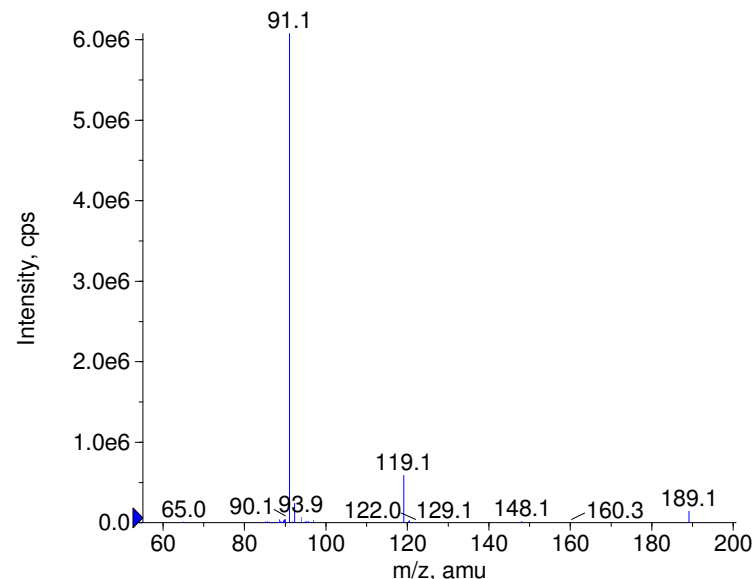
+ Fenproporex Prec(189.0) CE(50.0) RT(0.9)
