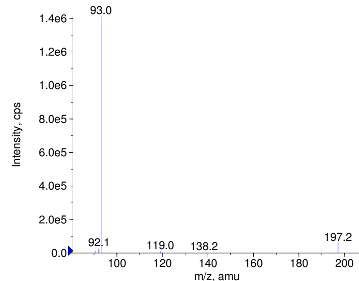
■ - Fenopropfen Prec(241.0) CE(-99.0) RT(1.0)
