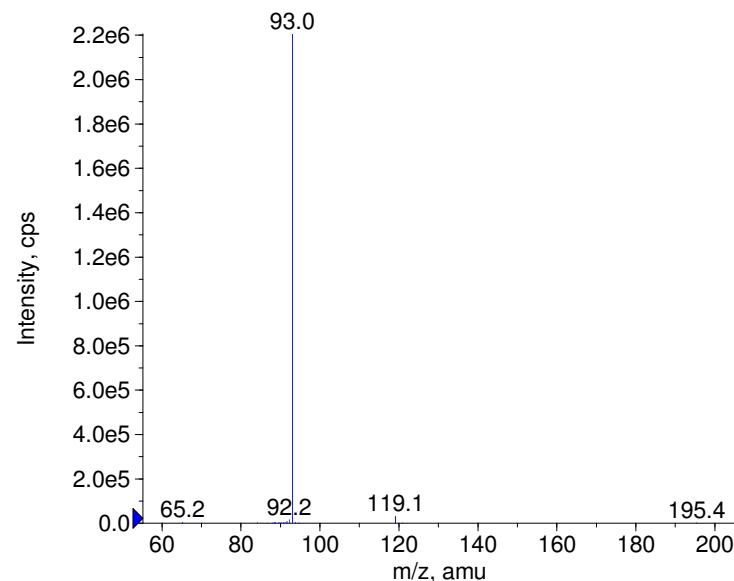
■ - Fenopropfen Prec(241.0) CE(-50.0) RT(1.0)
