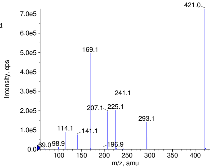
■ + Etofyllinclofibrate Prec(421.0) CE(50.0) RT(1.2)
