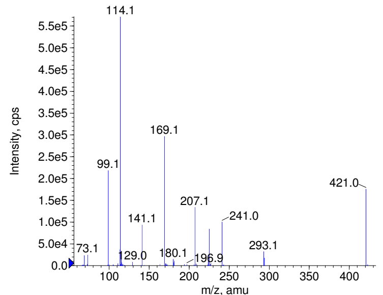
■ + Etofyllinclofibrate Prec(421.0) CE(99.0) RT(1.2)
