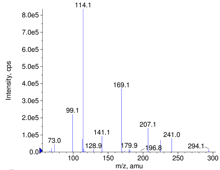
■ + Etofyllinclofibrate Prec(421.0) CE(99.0) RT(1.2)
