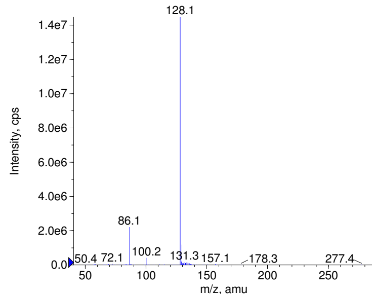
+ Etidocaine Prec(277.0) CE(99.0) RT(0.8)
