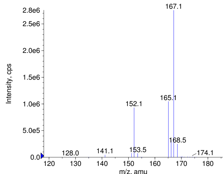
+ Ethylbenzhydramine Prec(284.0) CE(99.0) RT(0.9)
