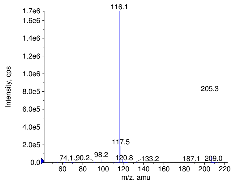
+ Ethambutol Prec(205.0) CE(50.0) RT(0.8)
