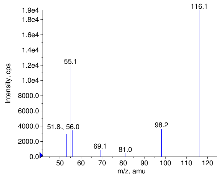
+ Ethambutol Prec(205.0) CE(50.0) RT(0.8)
