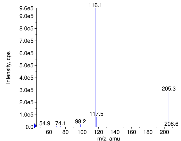
+ Ethambutol Prec(205.0) CE(99.0) RT(0.8)
