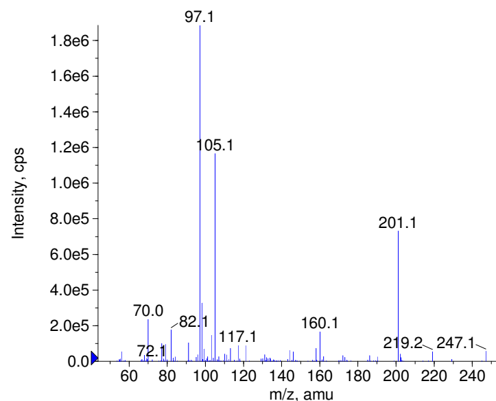
+ Eprazinone Prec(381.0) CE(50.0) RT(1.0)
