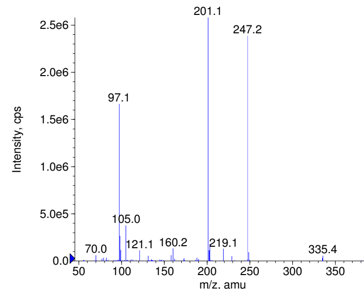
+ Eprazinone Prec(381.0) CE(99.0) RT(1.0)
