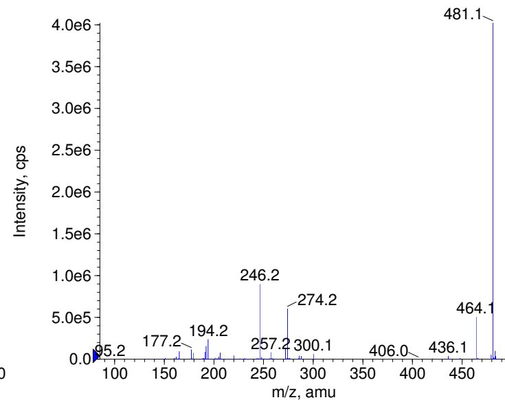
+ Emetine Prec(481.0) CE(99.0) RT(1.3)
