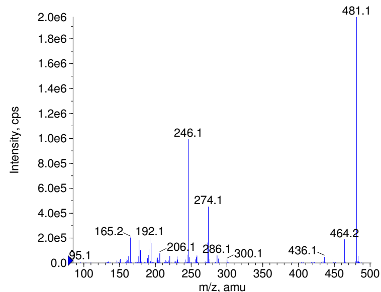
+ Emetine Prec(481.0) CE(99.0) RT(1.3)
