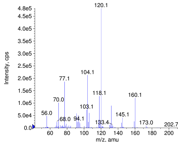
+ Dropropizine Prec(237.0) CE(50.0) RT(0.9)
