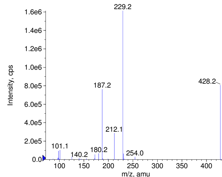
+ Dixyrazine Prec(428.0) CE(99.0) RT(0.9)
