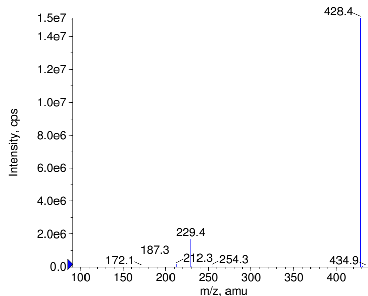
+ Dixyrazine Prec(428.0) CE(50.0) RT(0.9)
