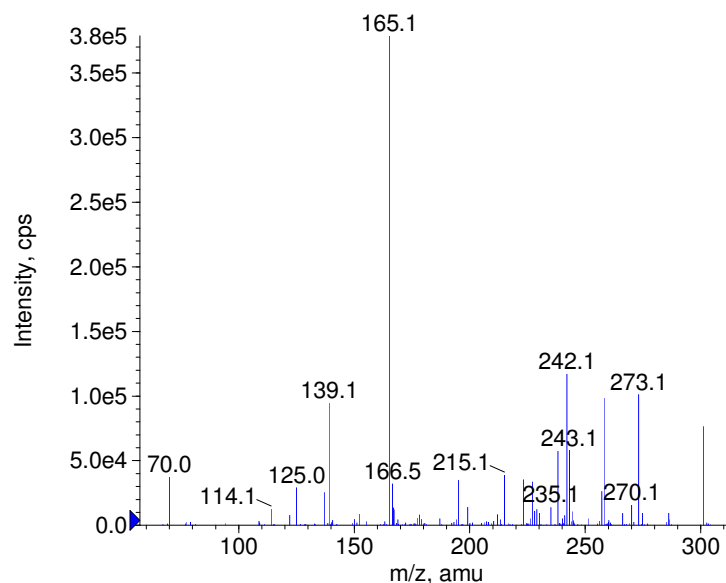
+ Dimethomorph Prec(388.0) CE(50.0) RT(1.0)
