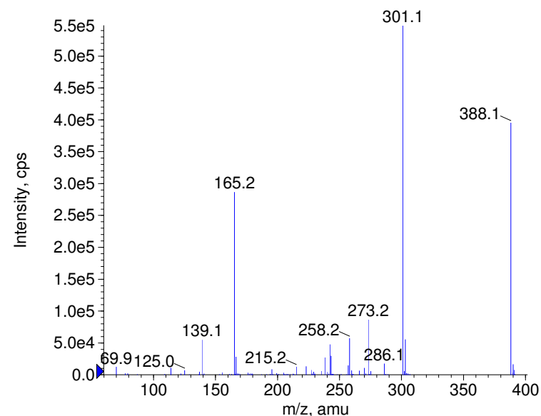
+ Dimethomorph Prec(388.0) CE(99.0) RT(1.0)
