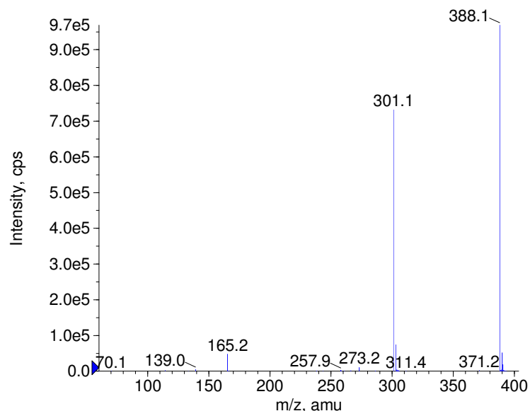
+ Dimethomorph Prec(388.0) CE(50.0) RT(1.0)
